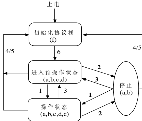
图 2.2 XGate-COP12 状态转换图
