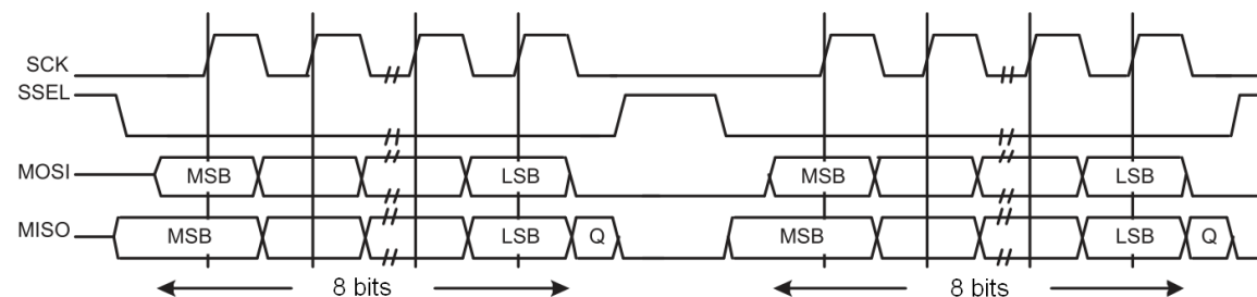
图 6.1 SPI 传输模式 0
