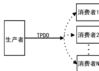
图 1.2 生产者消费者模型
