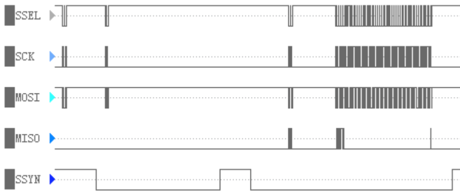
图 6.3 一次完整的 SPI 通信
