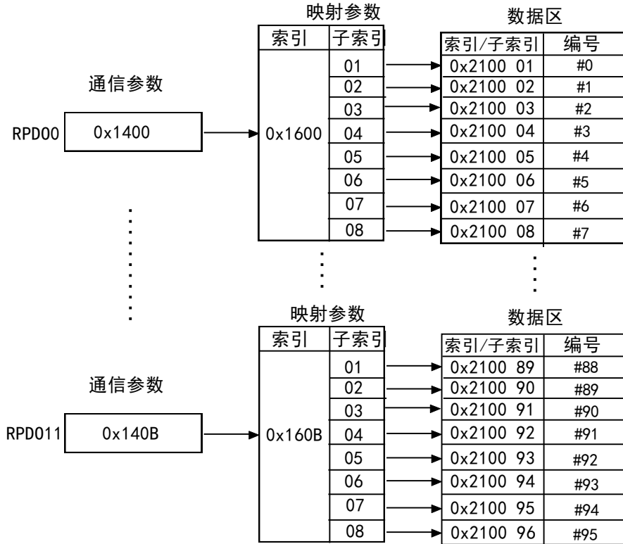
图 4.1 RPDO 映射关系
