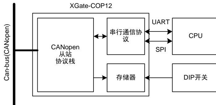
图 2.1 XGate-COP12 系统结构
