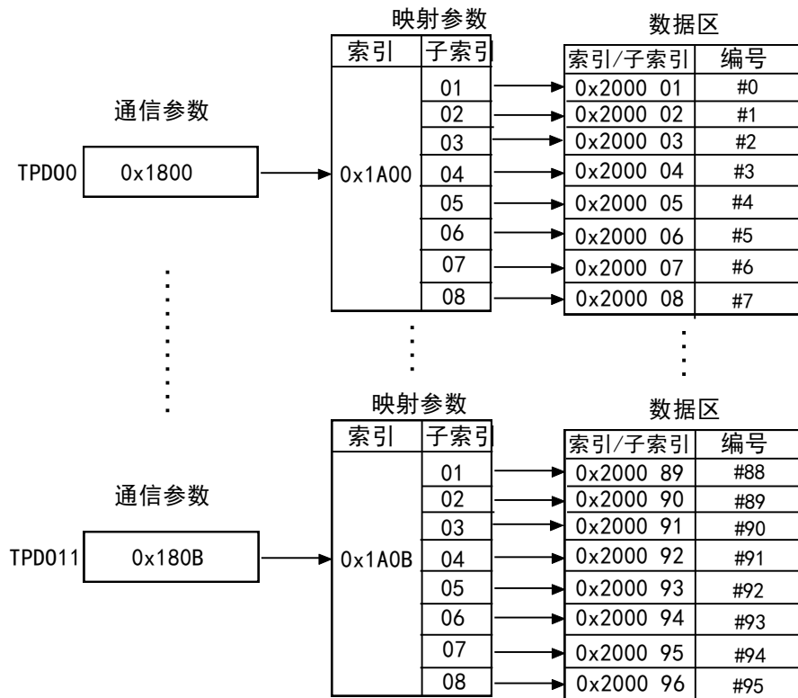
图 4.2 TPDO 映射关系
