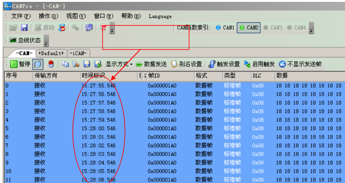
图 4.3 TPDO0 发送数据
