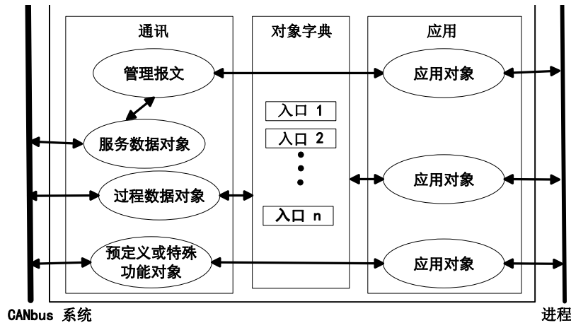
图 1.1 CANopen 设备结构
