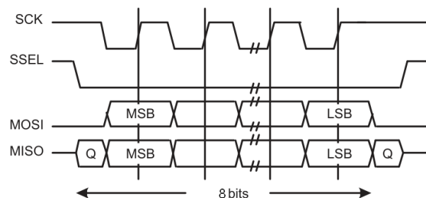
图 6.2 SPI 传输模式 3
