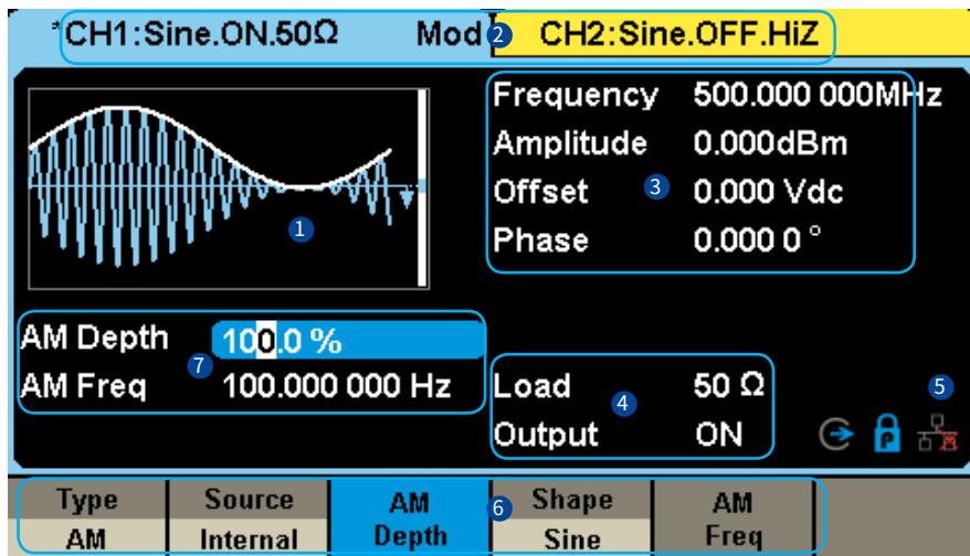
图 4 SDG6000X 触摸屏显示区
