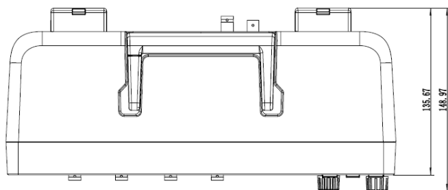
正视图
