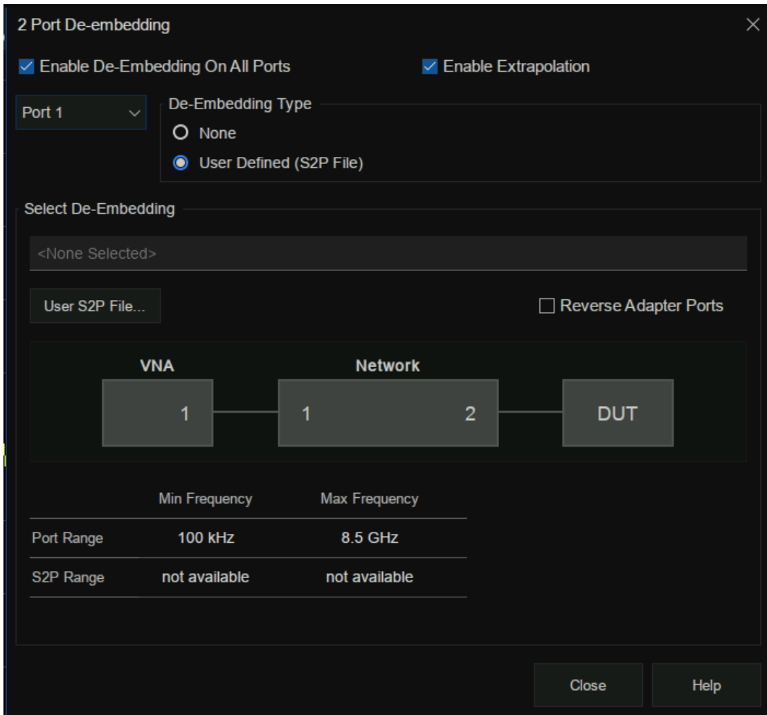
图 3-33 去嵌入界面
