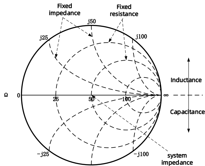
图 2-7 逆向史密斯圆图示意图
