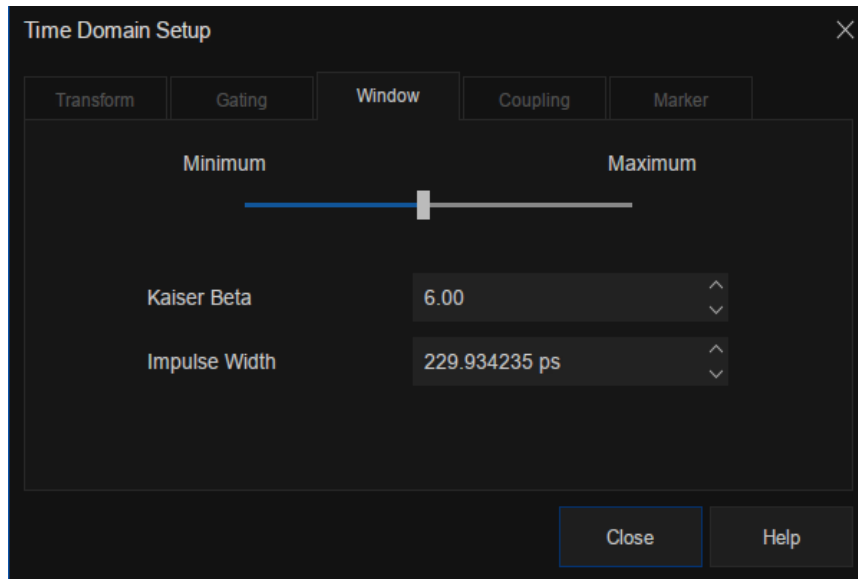
图 4-14 窗口设置
