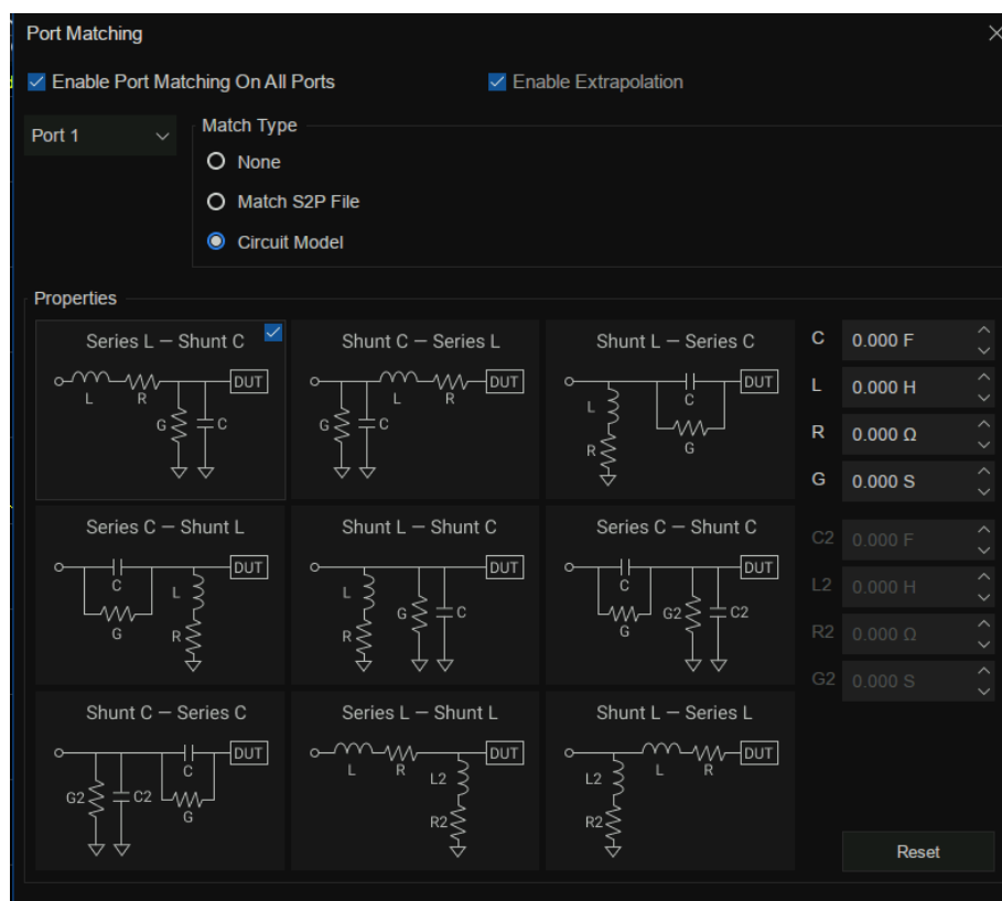
图 3-31 端口匹配
