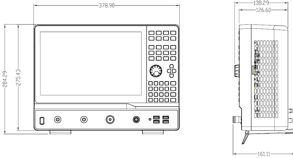
图 1-1 前视图和侧视图
