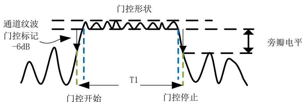
图 4-13 门控示意图
