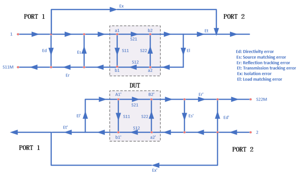
图 3-24 误差模型示意图
