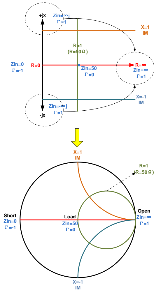
图 2-6 史密斯圆图示意图
