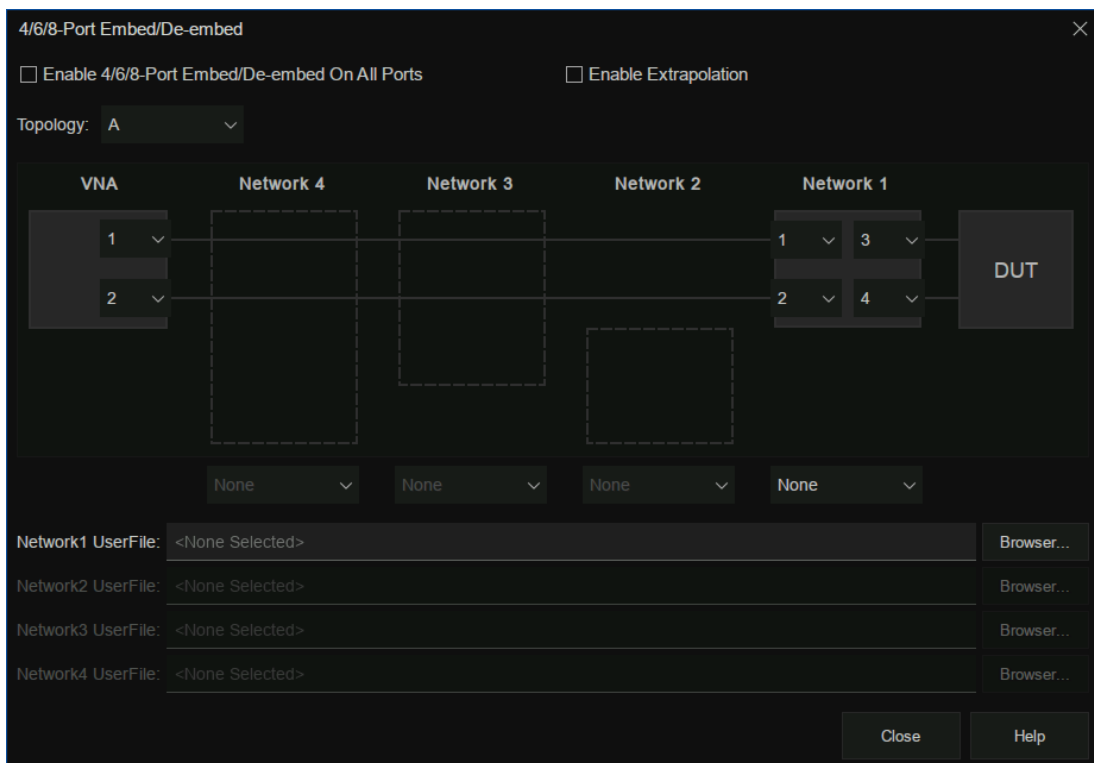
图 3-34 去嵌入界面
