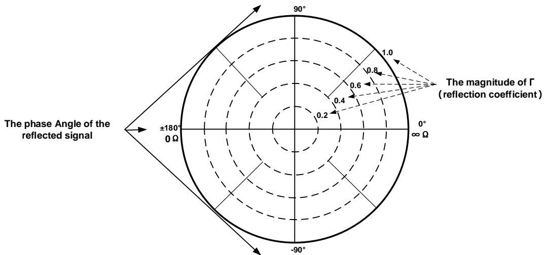
2-5 极坐标示意图
