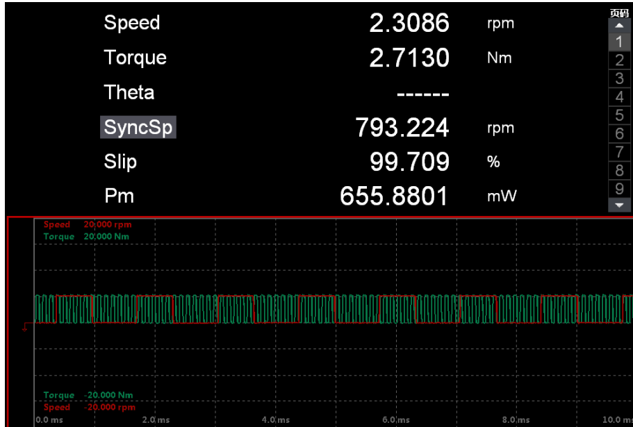
图 2.17 电机测量
