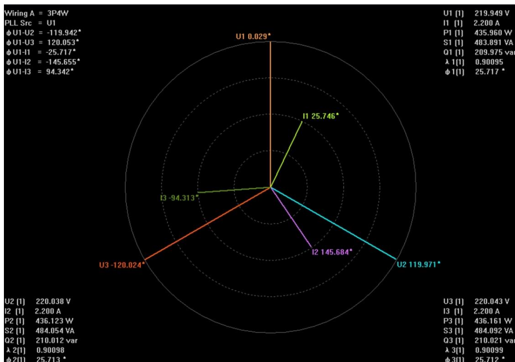
图 2.12 向量显示
