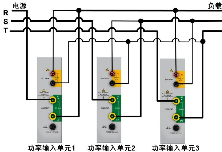
图 4.45 3P3W (3 电压 3 电流表法) 下功率分析仪接线示例
