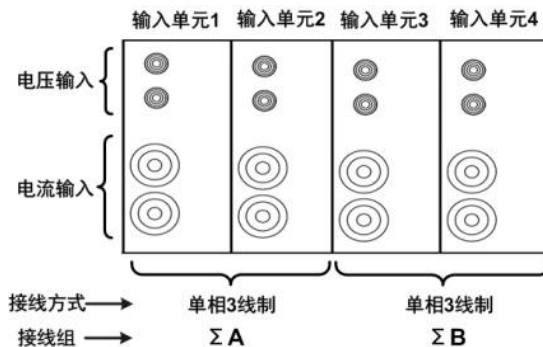
图 2.20 接线组
