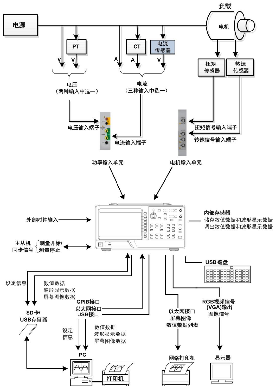
图 1.2 应用系统
