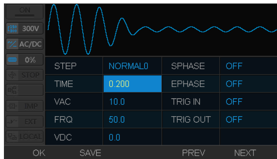
图 5.29 正常供电状态设置界面
