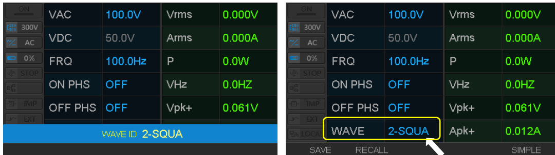
5.16 任意波形输出设置界面
