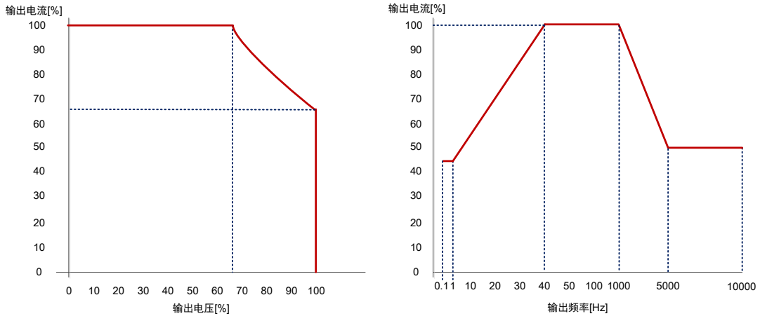
图 2.4 输出电压与输出频率允许输出电流范围
