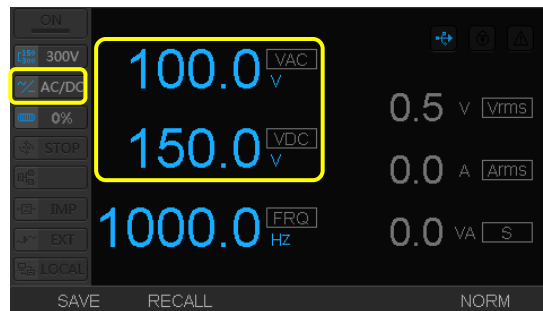
图 4.8 AC+DC 模式电压值设定
