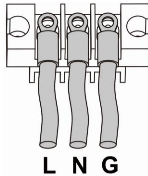
图 3.3 AC 端口接线
