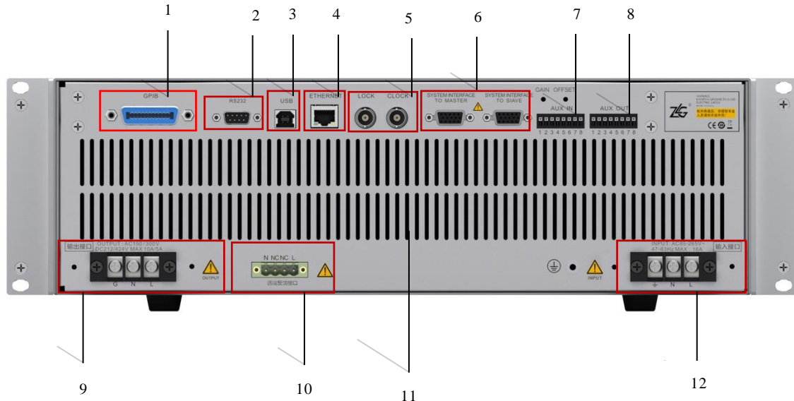
图 2.11 PWR1000L 后面板
