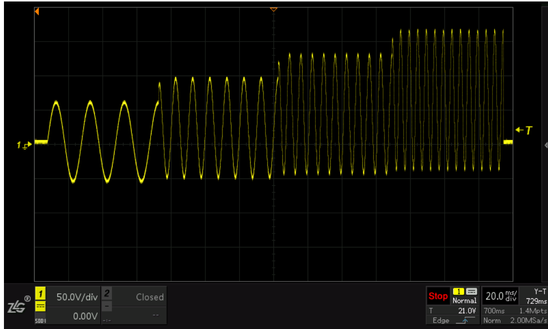
图 5.22 STEP 输出波形图
