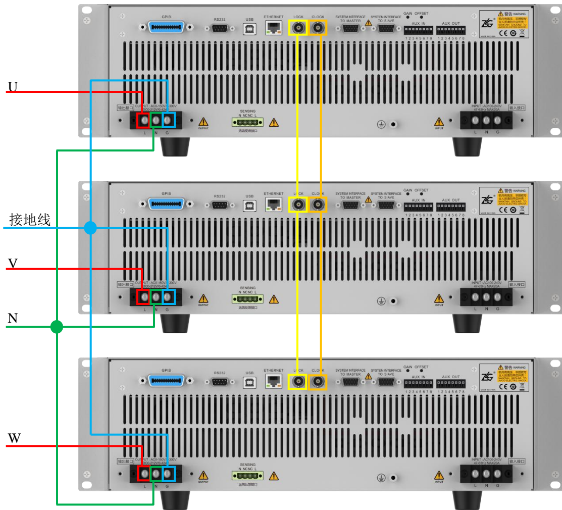
图 5.94 星形接法
