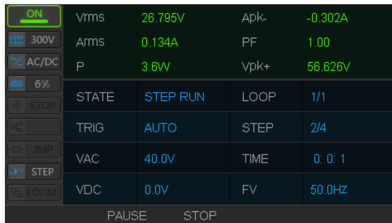
图 5.21 STEP 输出信息
