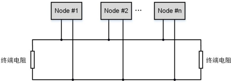
图 2.1 CAN-bus 网络拓扑结构
