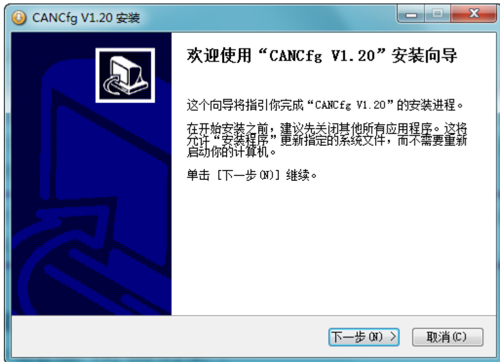
图 3.1 欢迎界面
