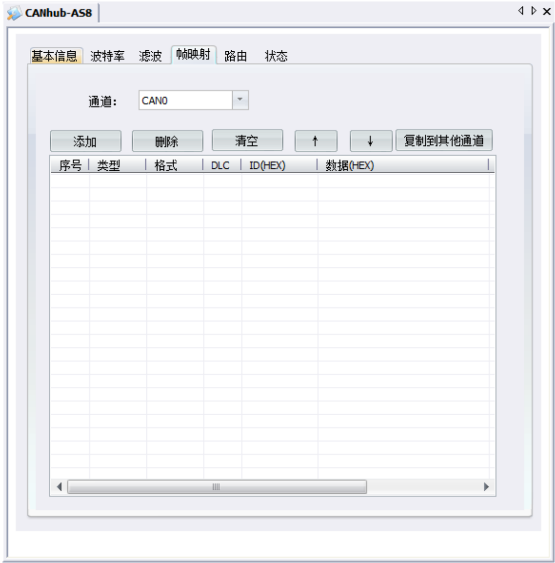
图 4.10 帧映射窗口
