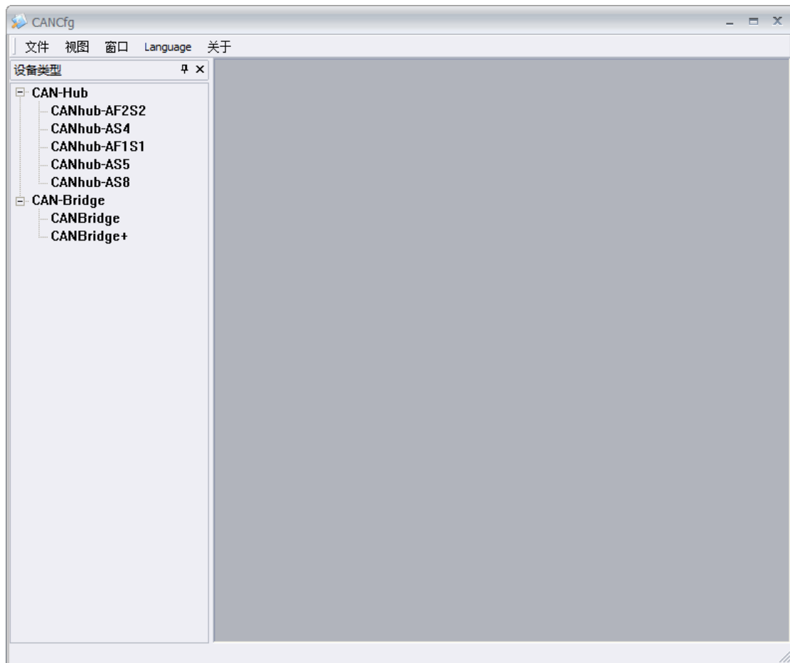
图 4.1CANCfg 运行界面
