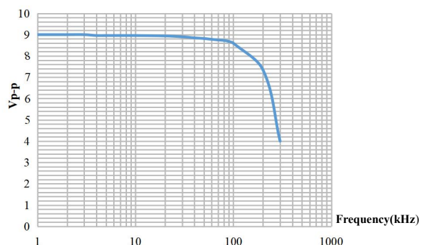
小信号幅频特性
