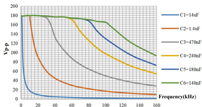
ATA-3080 容性负载曲线图
